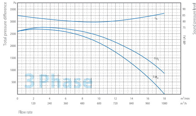
MAB-20A/T
