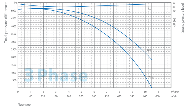
MAb-10D/T
