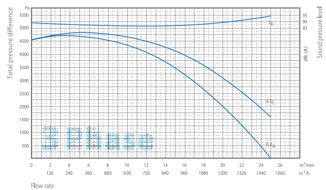
MAB-20D/T
