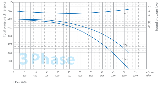
MAb-55B/T
