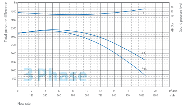
MAB-20B/T
